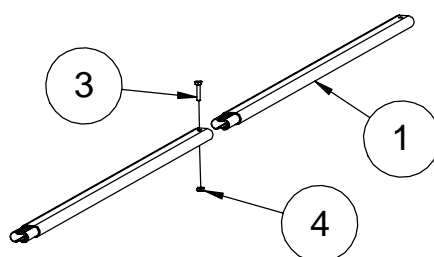
Vamzdžių prailginimas.
